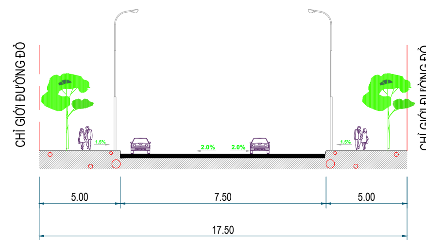
MẶT CẮT 1 - 1
