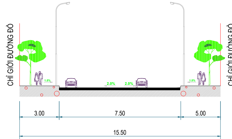
MẶT CẮT 2 - 2
