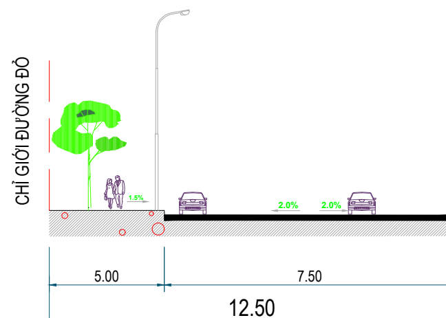
MẶT CẮT 4 - 4
