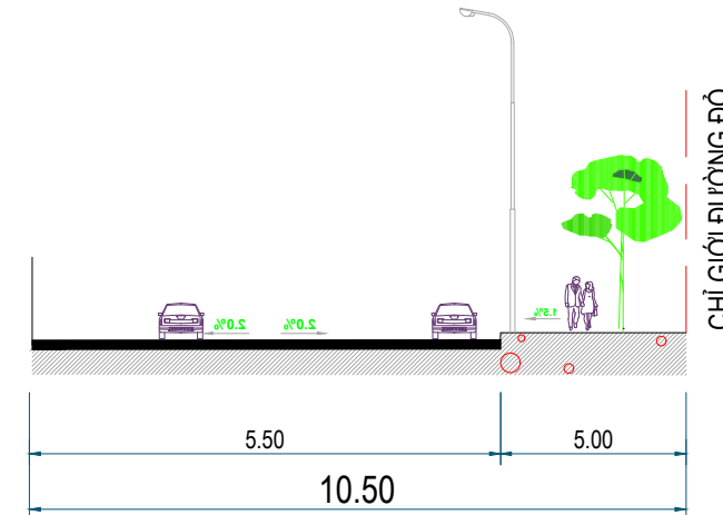
MẶT CẮT 3 - 3
